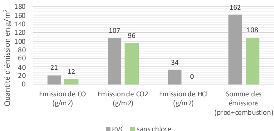
Analyse comparative des émissions de gaz entre les films PVC et sans chlore :
